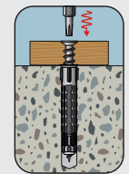
Zavrnuti vijak kroz rupu tako da bude u ravni s građevinskim elementom
